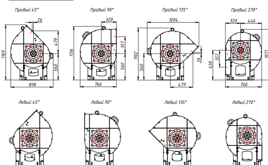
Индустриальный вентилятор BP 400 №4,5
