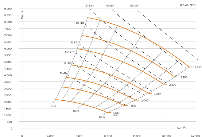
Индустриальный вентилятор BP 400 №7,1
