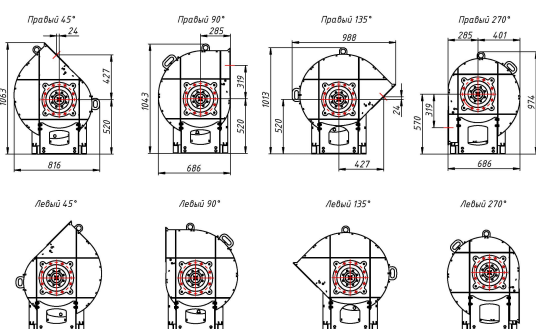
Индустриальный вентилятор BP 400 №4
