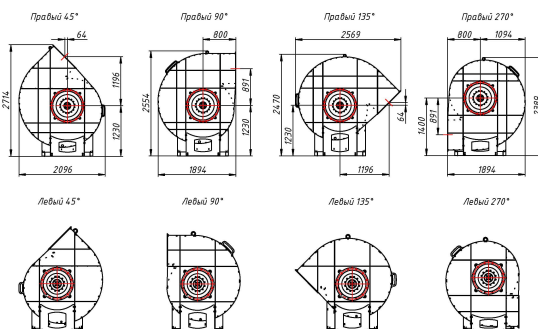
Индустриальный вентилятор BP 400 №11,2
