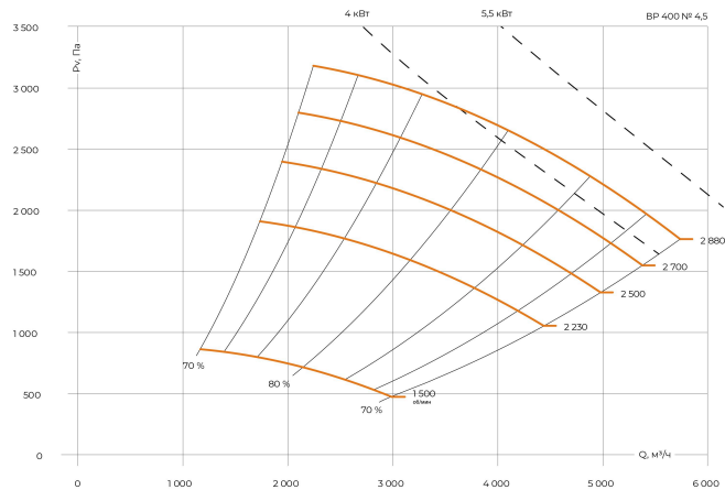
Индустриальный вентилятор BP 400 №4,5
