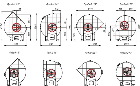
Индустриальный вентилятор BP 400 №10
