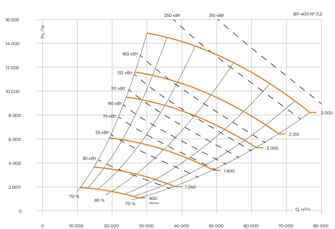
Индустриальный вентилятор BP 400 №11,2
