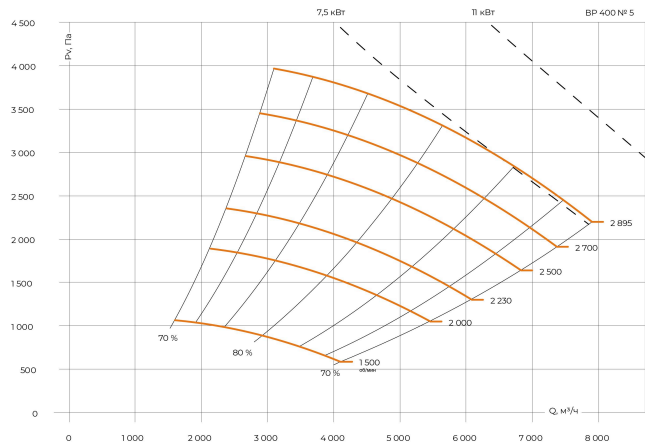
Индустриальный вентилятор BP 400 №5
