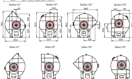
Индустриальный вентилятор BP 400 №8
