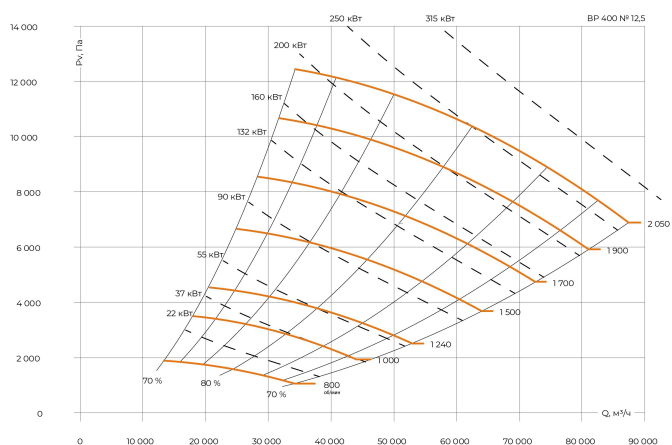
Индустриальный вентилятор BP 400 №12,5
