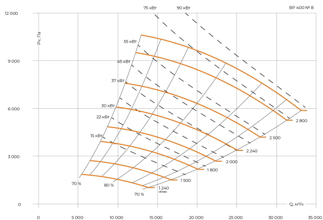
Индустриальный вентилятор BP 400 №8
