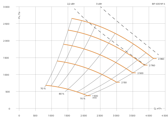
Индустриальный вентилятор BP 400 №4
