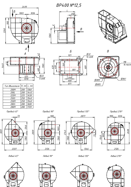
Индустриальный вентилятор BP 400 №12,5
