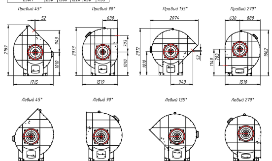
Индустриальный вентилятор BP 400 №9
