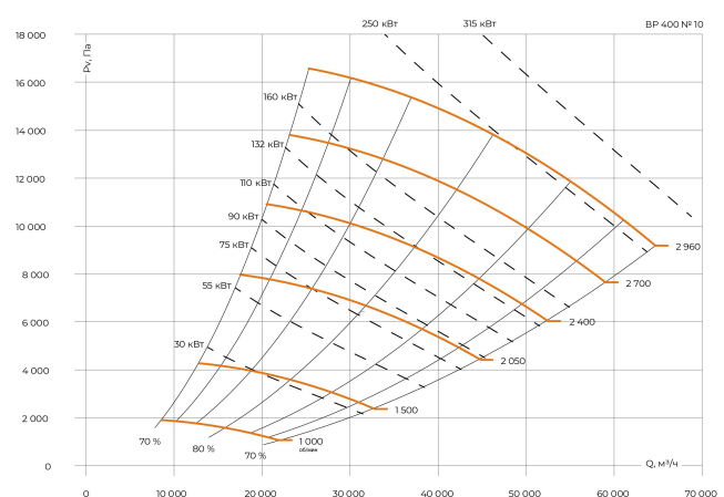
Индустриальный вентилятор BP 400 №10
