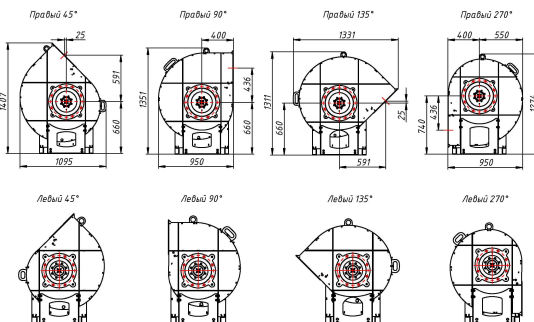
Индустриальный вентилятор BP 400 №5,6
