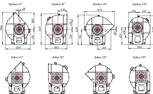
Индустриальный вентилятор BP 400 №6,3
