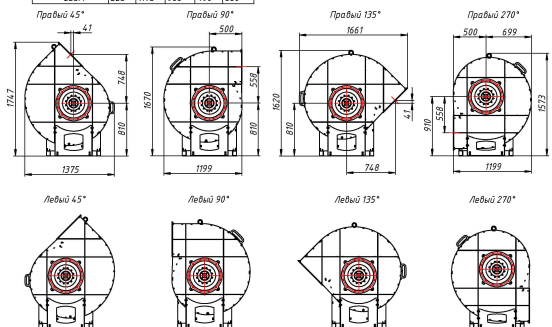
Индустриальный вентилятор BP 400 №7,1
