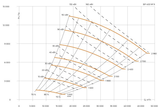
Индустриальный вентилятор BP 400 №9
