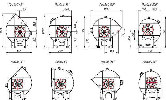
Индустриальный вентилятор BP 400 №5
