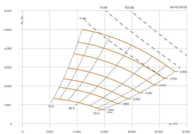
Индустриальный вентилятор BP 400 №5,6
