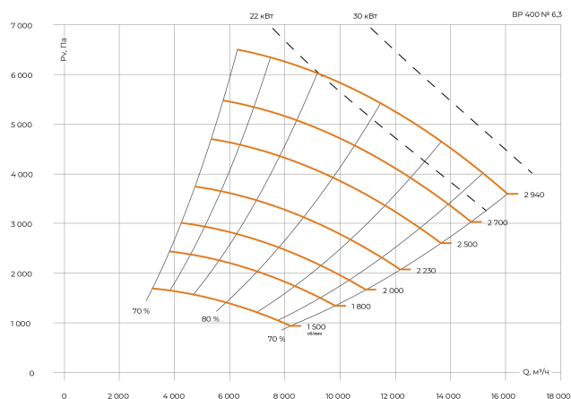
Индустриальный вентилятор BP 400 №6,3
